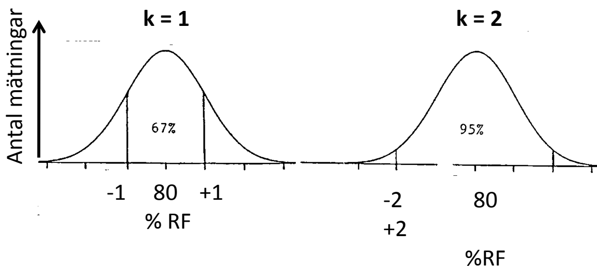
Figur 27.4. Täckningsfaktorns inverkan på mätosäkerheten
